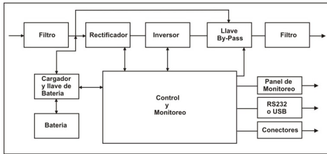
Fig.1. Diagrama en bloques del UPS
